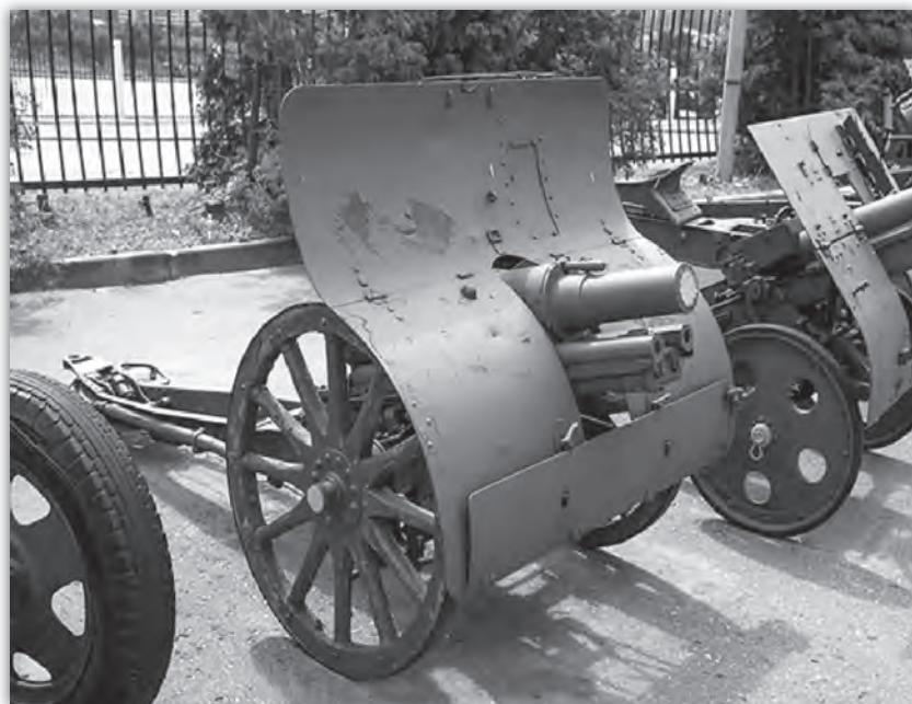
3-х дюймовая горная пушка системы Шнейдера была принята на вооружение Высочайшим повелением от 26 февраля 1909 года
