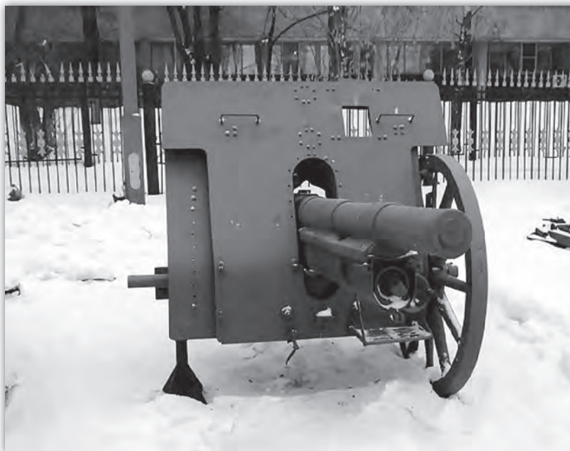
Вторая японская пушка – 77 мм полевая пушка образца 1925 года
